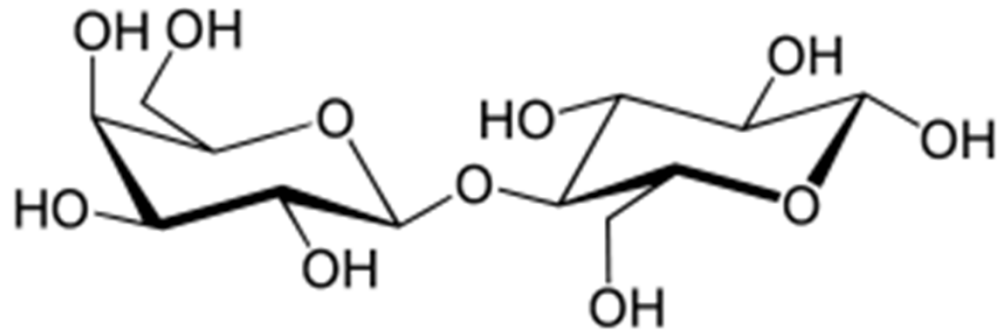
Lactose
