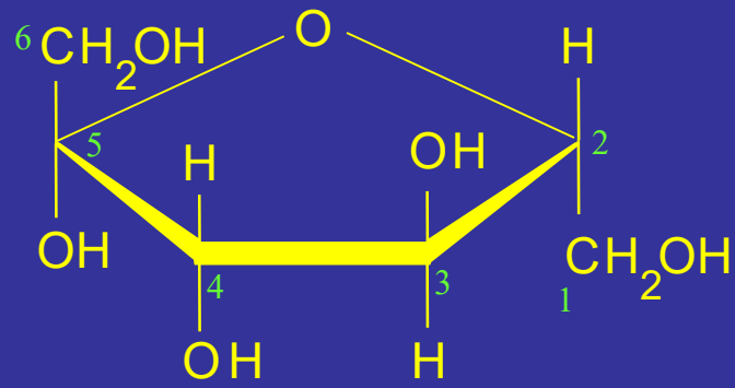
\beta -D-fructose
