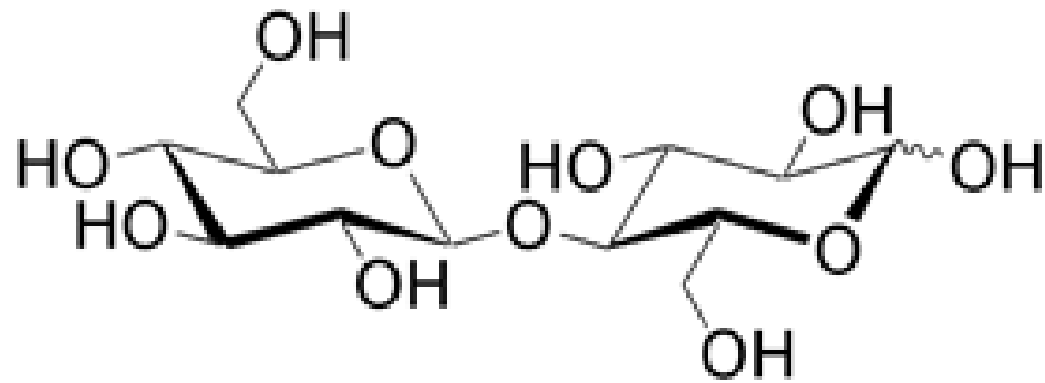
Cellobiose
